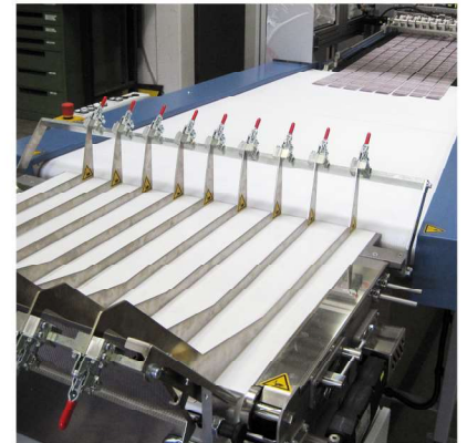
Auslagevariante Spreizband mit Schachtauslage SB 810
